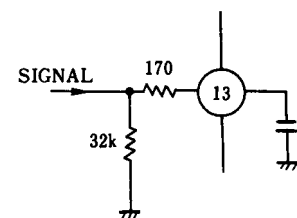
⟨RSSI Output⟩
